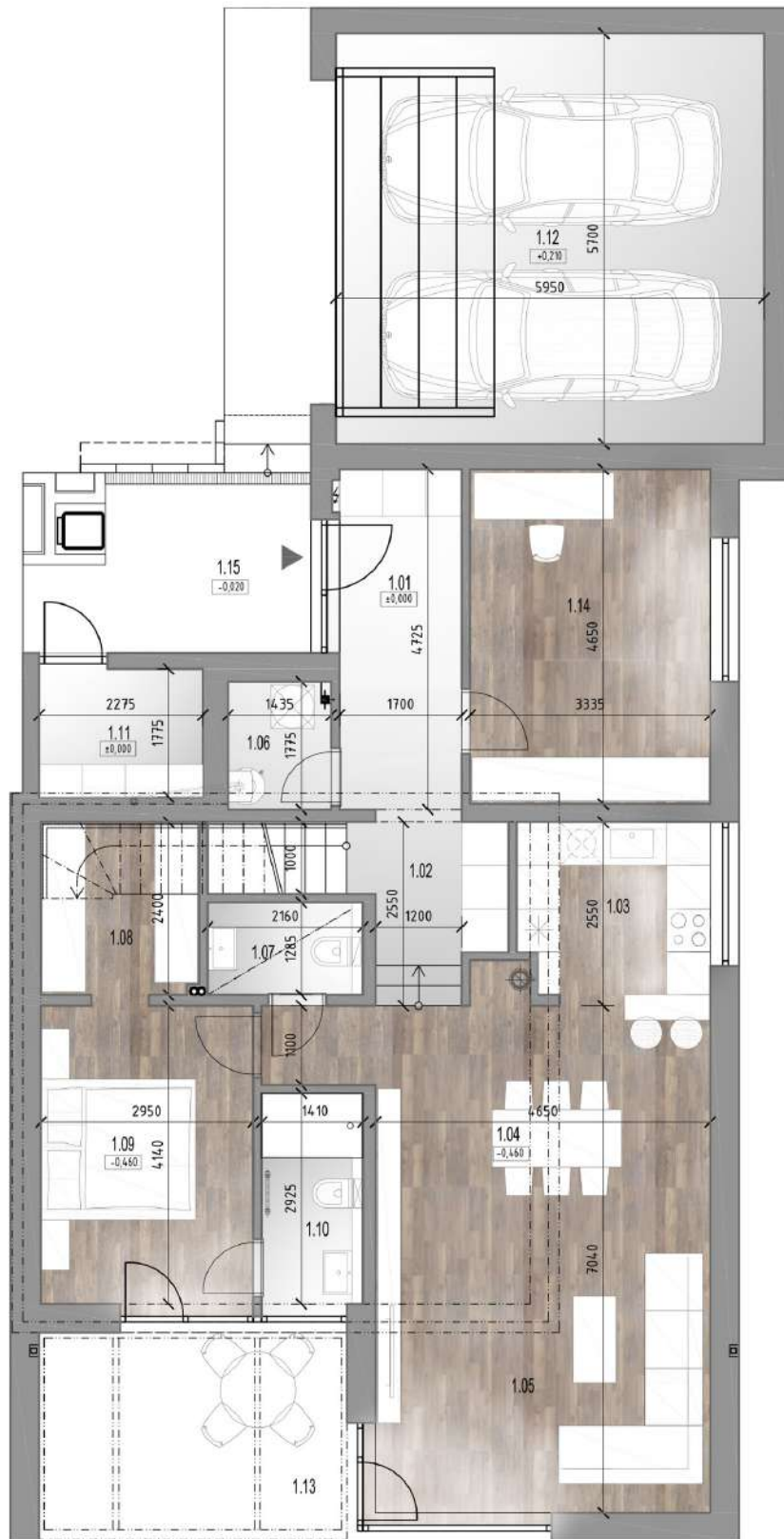
1. NADZEMNÉ PODLAŽIE
